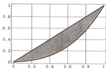
Obrázek 3.10: Lorenzova křivka a míra nerovnosti
