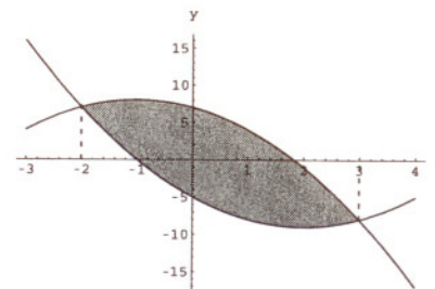
Obrázek 3.8: Plocha ohraničená grafy funkcí
