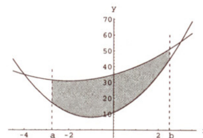
Obrázek 3.6: Plocha ohraničená grafy funkcí a přímkami x = a a x = b
