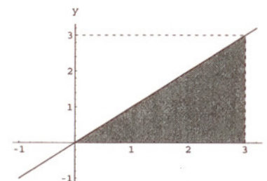
Obrázek 3.3: Plocha ohraničená grafem funkce f(x) = x , osou x a přímkou x = 3
