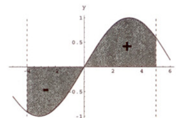
Obrázek 3.2: Rozložení intervalu \langle a, b \rangle na
