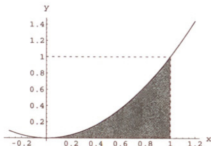
Obrázek 3.4: Plocha ohraničená grafem funkce f(x) = x^2 , osou x a přímkou x = 1
