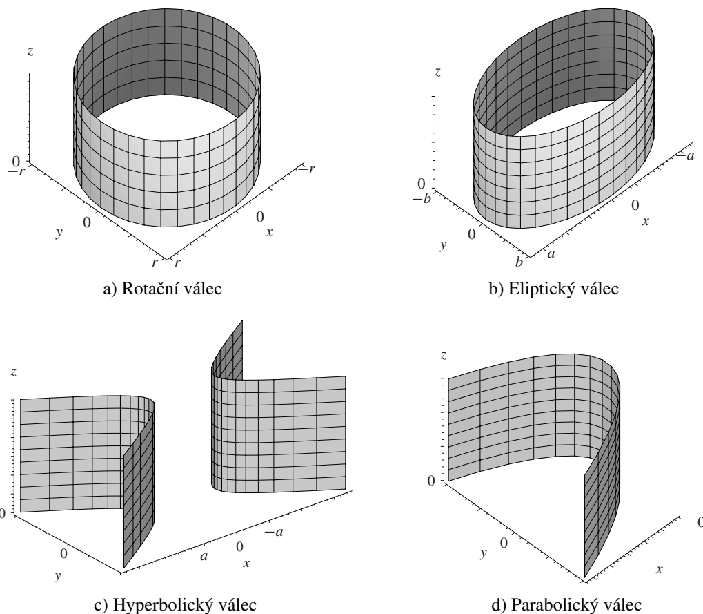
Obr. 9.3: Kvadratické válce
