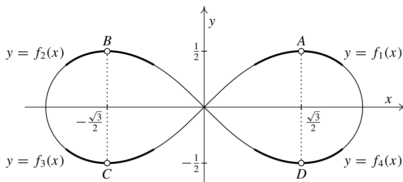
Obr. 7.4: Bernoulliiova lemniskáta
