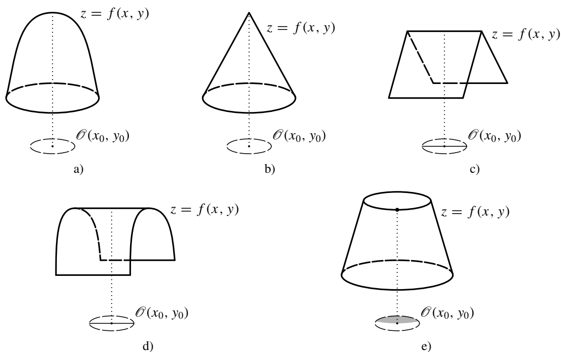
Obr. 5.1: Lokální maxima
