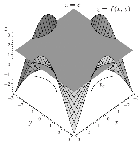
Obr. 1.7: Vrstevnice
